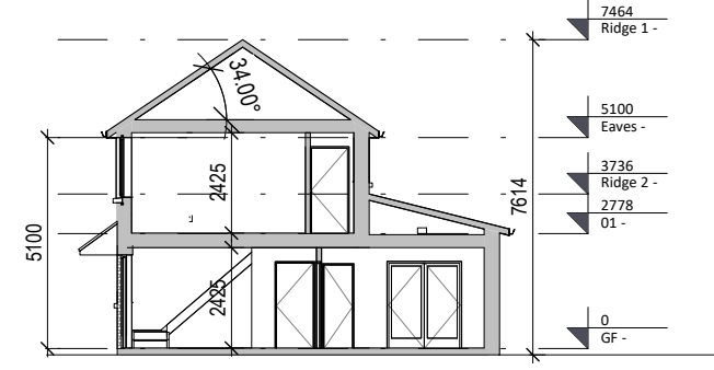
③ Section A-A 1 : 200
